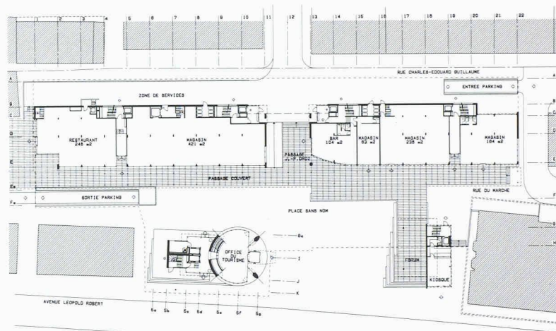
Plan d'ensemble
