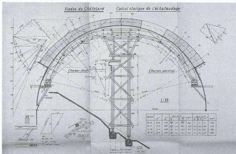
Viaduc du Châtelard, voie ferrée Lausanne-Berne: remplacement de l'ouvrage métallique par un viaduc en maçonnerie (1924-1925). Calculs statiques des échafaudages (voir également page de couverture). Document ACM, Fonds A. Bühler
