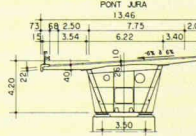
COUPE TRANSVERSALE
