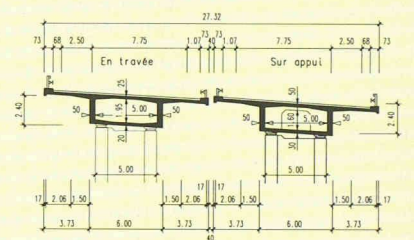
COUPE TYPE Tabliers exécutés en encoberlement (axes 13 à 18)
