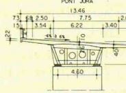
COUPE TRANSVERSALE
