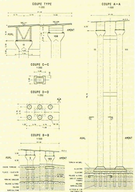
COUPE TYPE Tabliers exécutés sur cintres (axes 0 à 13 et 18 - 19)
