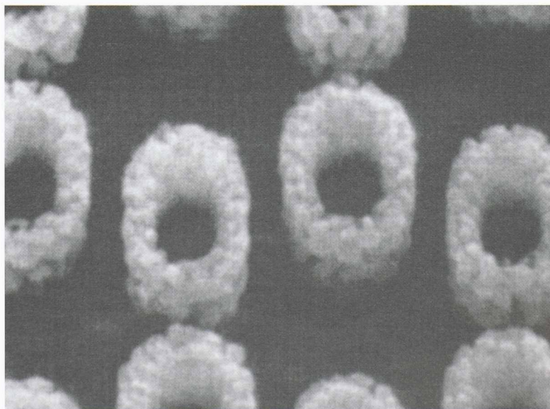
Fig. 5. — Photo de condensateurs HSG tirée de l'article de Kinam Kim et al., IEEE Transactions on Electron Devices , vol. 45, no. 3, mars 1998
