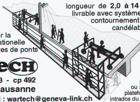
"CROC" avec train de roulement à emprise minimale sur les bords de la chaussée du pont
