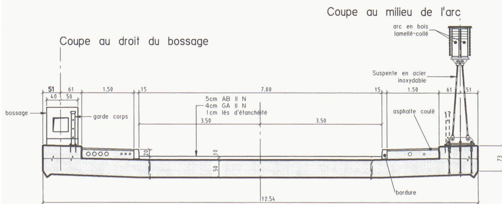
Fig. 5.- Coupes transversales
