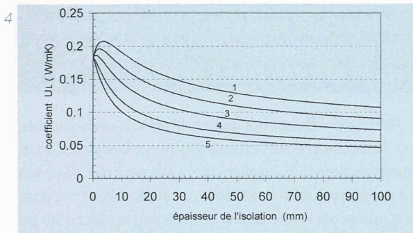
Coefficient de déperdition thermique linéaire en fonction de l'épaisseur d'isolation pour conduite en PVC de diamètre d_i = 5 et d_e = 8 mm, h_e = 8 W/m 2 K 1: \lambda = 0,06 W/mK, e_c = 12,5 mm 2: \lambda = 0,05 W/mK, e_c = 6,5 mm 3: \lambda = 0,04 W/mK, e_c = 2,5 mm 4: \lambda = 0,03 W/mK, e_c = 0 mm 5: \lambda = 0,025 W/mK, e_c = 0 mm
