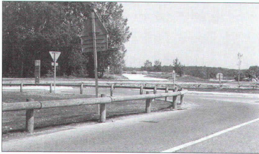
Glissières de sécurité mixtes bois-métal
