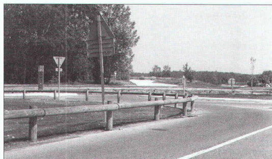
Glissières de sécurité mixtes bois-métal
