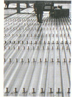
Tôle profilée (Photo Michel Crisinel, Lausanne)
