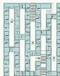
Plan type du projet « Upsidetown », lauréat du concours EUROPAN 7, site de Fribourg (Document Roland Stutz, Martin Bruhin, Ruben Daluz Gonzalvo)
