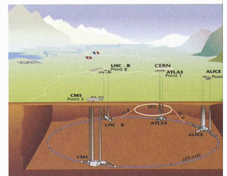
Fig. 3 : Schéma des installations pour le LHC (Source : CERN)
