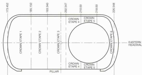
Exécution des plans d'armature de la caverne principale
