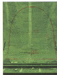
Profil de perçement transversal, tunnel de base du Gothard (Photo Milo Keller, ECAL)
