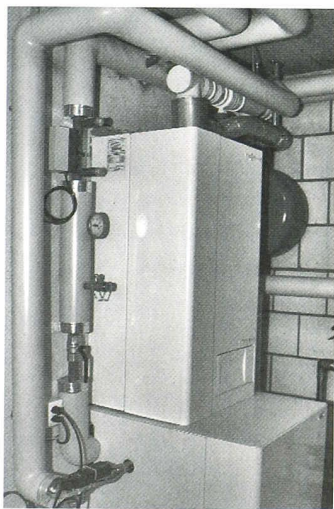
Parmi les chaudières à mazout à condensation existent aussi des chaudières murales.
