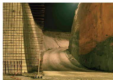
Rampe du chantier m2 à la Sallaz, janvier 2006 (Photo Léonore BaudfECAL)
