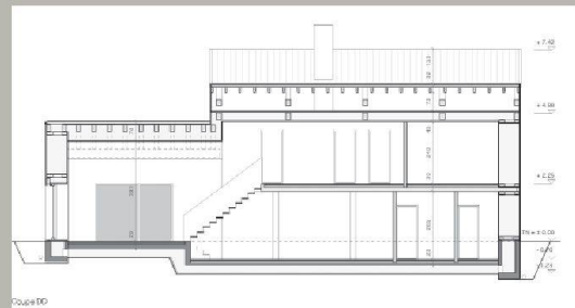
Coupes
