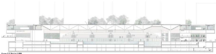
Coupe C-C Plaine 1:500
