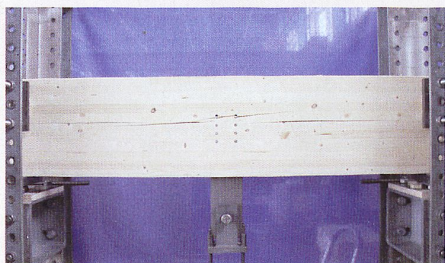
Fissuration d'une poutre : rupture en traction perpendiculaire d'un assemblage transversal avec des broches sollicitées perpendiculairement au fil – banc d'essais et éprouvette de l'EPF Zurich. (Photo Robert Jockwer, IBK de l'EPFZ)
