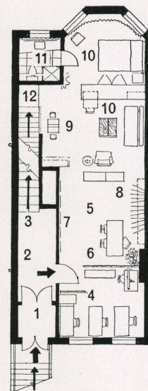
Grundriß der oberen Verkaufsräume Plan des salles de vente supérieures Plan of the upper floor salesrooms
