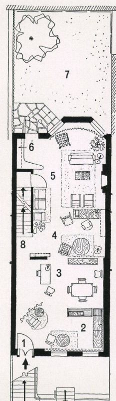
Grundriß der unteren Verkaufsräume Plan des salles de vente inférieures Plan of the ground floor salesrooms
