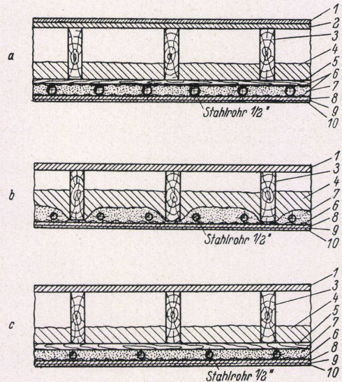
Abb. 1b Rohrdeckenheizungen im Verputz an drei Holzbalkendecken dargestellt
