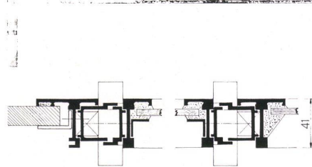
Abb. 4 Horizontalschnitt durch Schwingflügelpartie vom Industriefenster, System «Vohland & Bär» (Typ VB 41/J), Einfachverglasung. Fabrikation: Vohland & Bär AG., Riehen/ Basel.
