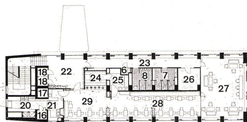
Normalgeschoß-Grundriß 1:300. Plan d'un étage normal. Typical floor plan.
