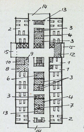
5 Thurgauisches Kantonsspital Münsterlingen (Skizze 1958), Architekten: A. Muggler und E. F. Burckhardt BSA/SIA, Zürich. Doppelbündiger Grundriß mit Ost- und Westzimmer, zwei Drittel der 50 Betten südlich und ein Drittel nördlich des Verkehrszentrums, mittlere Nebenräume in aufgelockerter Form, allgemeine Nebenräume dem Verkehrszentrum angeschlossen. Dieser Grundriß macht sich die hervorragende Aussichtslage der Situation Münsterlingen nach Norden zu Nutzen.
