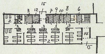
3 Kreisspital Bülach, Architekt E. Schindler BSA/SIA, Zürich, Erweiterungsprojekt. Im Prinzip klassischer Grundriss wie Winterthur, jedoch mit Heranziehen der wichtigsten Nebenräume wie Ausguß, WC, Blumenräume an die Bettenabteilung.
