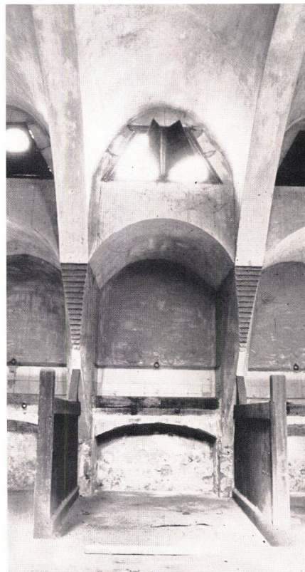
7–10 Gewölbekonstruktion eines Stallgebäudes in der Finca Güell in Barcelona 1887. Reine Steinkonstruktion, deren Abmessungen auf das Äußerste reduziert sind. Die außen sichtbaren Tonnen erinnern schon an Schalenkonstruktionen, wie sie heute verwendet werden; die Tonnen wirken jedoch hier als Gewölbe, da sie aus Stein bestehen und am Rand voll durch scheibenartige Bögen unterstützt sind. Die Lasten der Tonnen G_R und G_L (Abb. 7) bilden die Resultierenden \Sigma G_V , die als Stützlínien innerhalb des Bogens in die Fundamente geleitet werden. Die für die damalige Zeit kühne Konstruktion und die Form bilden eine untrennbare Einheit.
