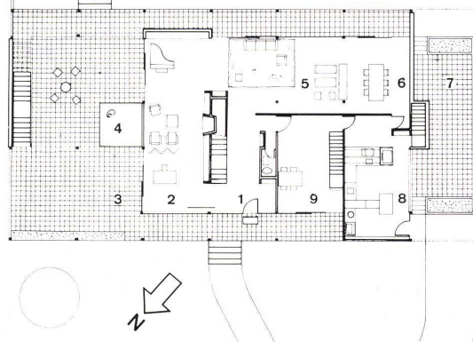
3 Lageplan und Grundriß Erdgeschoß 1 : 350. Plan de situation et plan de rez-de-chaussée. Site plan and plan of the ground floor.
