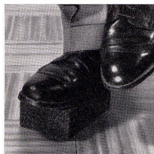
Stark und starr – Legen Sie Ihr FOAMGLAS-Muster auf den Boden und stehen Sie darauf: Es wird nicht zusammengedrückt, denn seine Druckfestigkeit ist 7 kg/cm 2 . FOAMGLAS ist auch formbeständig und kann weder schwinden noch quellen.
