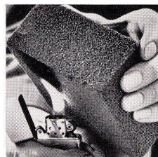
Unbrennbar, anorganisch – Halten Sie das Muster gegen eine Flamme: FOAMGLAS brennt nicht – ein bedeutender Sicherheitsfaktor für alle Gebäude. FOAMGLAS kann aber auch nicht verrotten und ist beständig gegen gewöhnliche Säuren und saure Dämpfe.
