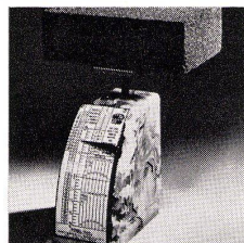
Leicht – Wenn Sie Ihr FOAMGLAS-Muster in die Hand nehmen, fühlen Sie sofort, wie leicht dieses Material ist. Wiegen Sie nach: Ein Kubikmeter FOAMGLAS wiegt nur 144 kg.
