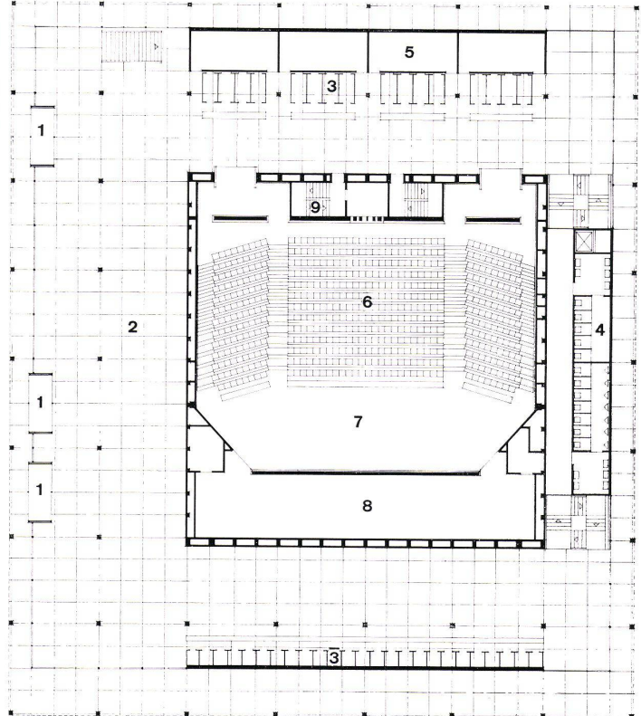
3 Foyergeschoß mit Physiksaal / Etage du foyer avec salle de physique / Foyer level with physics room 1:500
