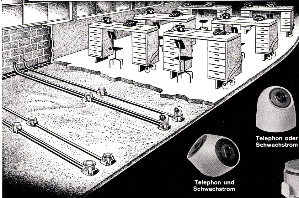
Bodendose mit Regulierring zur bodenbündigen Einstellung des Dosendeckels
