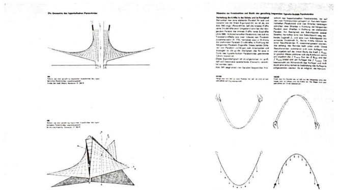
3 Doppelseite aus der allgemeinen Konstruktionsanalyse und Schalenstatik im Abschnitt «Zweifach gekrümmte Schalen mit gegensinnigen Hauptkrümmungen».
