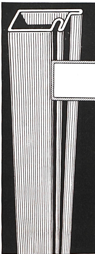
Kittleiste aus Hart-PVC Dichtung aus Kunststoff
