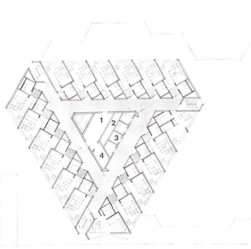
5 17. Geschoß des projektierten Hotels 1:500. 17ème étage de l'hôtel projeté. 17th floor of planned hotel. 1 Wäschelager / Linges et literie / Linen 2 Installationsschacht / Canal d'installations / Installations shaft 3 Personenlift / Ascenseur / Passenger lift 4 Warenlift / Monte-charge / Freight lift
