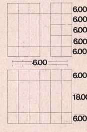
4 Konstruktives System 1:600. Système constructif. Construction system. Werkstatt 1836 m 2 / Atelier / Workshop Ersatzteillager 720 m 2 / Magasin des pièces de rechange / Spare parts stores Büro 176 m 2 / Bureau / Office Ausstellungsfläche 376 m 2 / Surface d'exposition / Display area Verkehrswege, Grünanlagen und Abstellplätze 1948 m 2 / Chemins de circulation, surfaces vertes et places de débarras / Communication routes, green areas and parking sites Grundstücksgröße 62x80 m 2 = 4960 m 2 / Dimensions du terrain à bâtir / Site area Überbaute Fläche 3012 m 2 / Surface bâtie / Built over area
