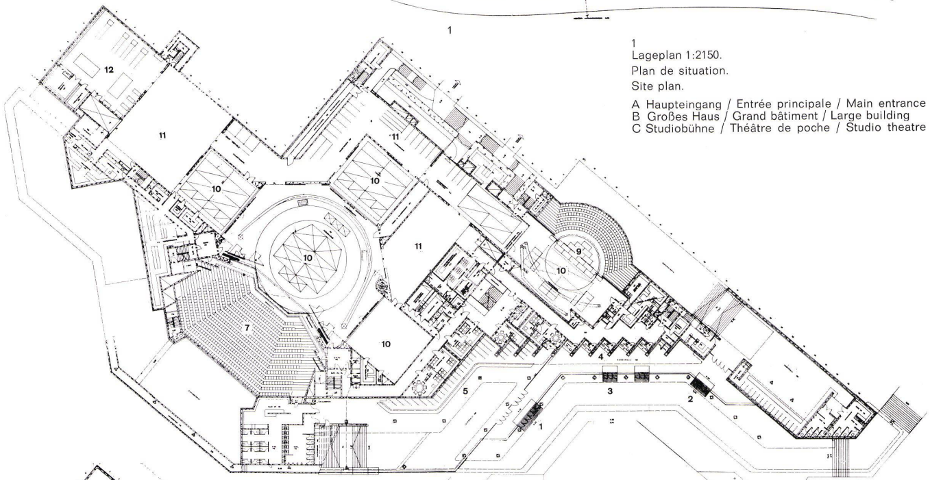
2 Erdgeschoß 1:900. Rez-de-chaussée.
