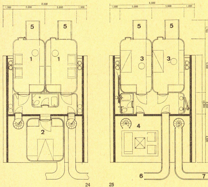
24 Grundriß einer Familieneinheit, unteres Geschoß 1:200.
