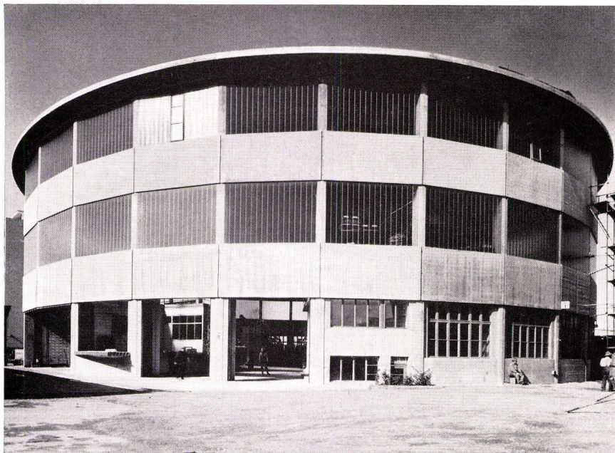
Rundhalle System Züblin MuttENZ BL
