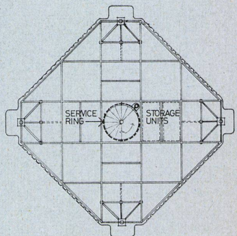
7 Strukturplan.
