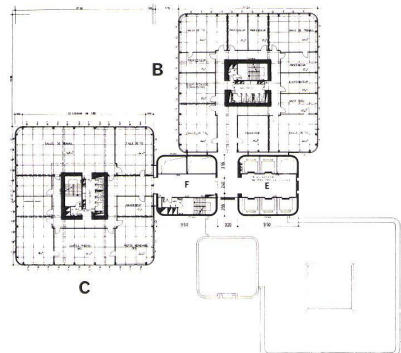
11 Grundriß 11. Obergeschoß 1:1000. Plan du 11ème étage. Plan of 11th floor.
