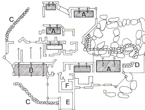
Funktionsschema. Schéma fonctionnel. Functional diagram.
