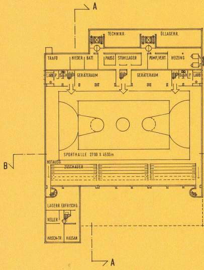
KELLERGESCHOSS
