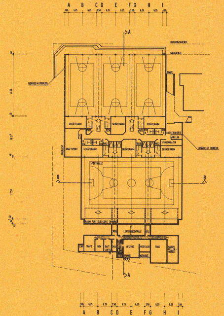
SPORTHALLE BRINKMANNSTRASSE GRUNDRISS UNTERGESCHOSS
