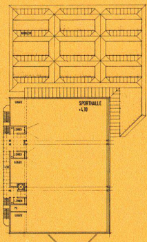
1.OG
