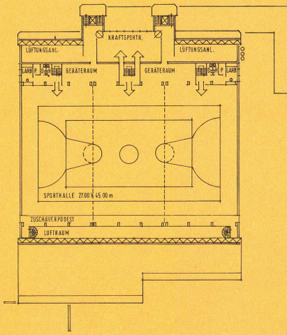
2. OBERGESCHOSS
