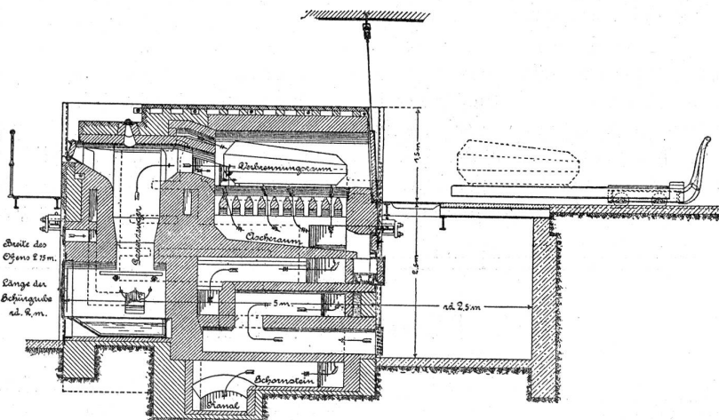
Längsschnitt der Ofenanlagen eines Krematoriums.
