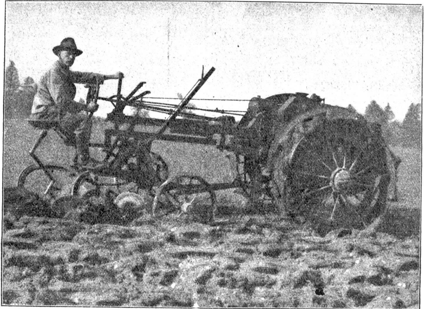
Motorpflug (amerikanisches System), angekauft von der eidgenössischen Brotkommission, zurzeit im Betrieb auf dem Waffenplatz Kloten.
