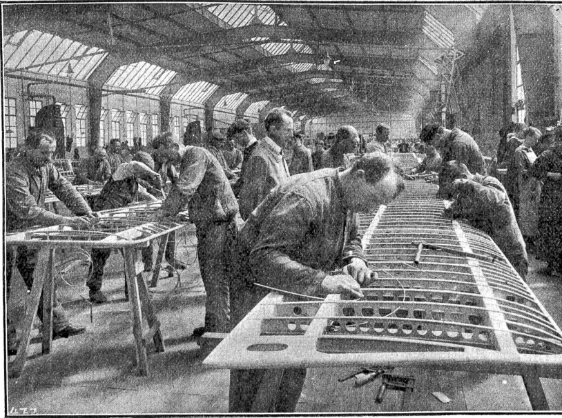
In einer deutschen Flugzeugfabrik: Verspannarbeiten an den Cragflächen. (Man sieht das Gerippe der Cragflächen ohne Stoffbekleidung.)
