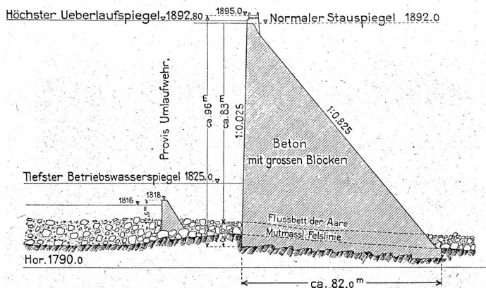
Querschnitt der Grimselpferre. — Maßstab 1:2000.
