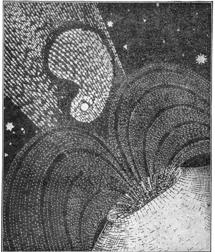
Die Gigantsternexplosion.
