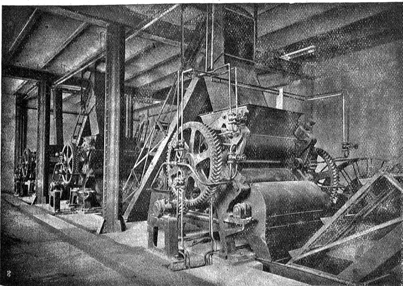
Abb. 4. Kalandier; Herstellung von Granit- und Jaspé-Linoleum.
