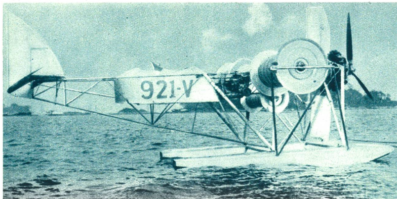
Amerikanische Erfindung: Flügelloses Flugzeug.
