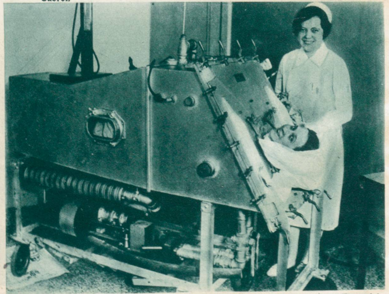
Bett in einen luftdichten Behälter gelegt, wobei nur der Kopf herausragt. Eine elek- trische Pumpe zieht dann die Luft aus dem Behälter, ungefähr 15mal jede Minute, und da jedesmal der Luftdruck in dieser Weise vermindert wird, müssen die Lungen des Kranken sich ausdehnen, ob er will oder nicht. Phot. Keystone.
