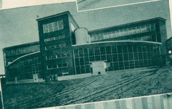
Rechts: Speicher- Kraftwerk Herdecke (Deutschland), aus- gerüstet mit drei Sulzer-Speicher- pumpen von je 12,300 Liter pro Se- kunde, 163 Meter Förderhöhe und 33,000 Pferdestär- ken Kraftbedarf. Phot. Gebr. Sulzer A.-G., Winterthur.
