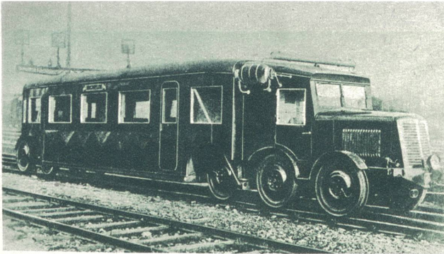
Das erste Schienenauto fährt durch die Schweiz, von Genf via Buchs, nach der Tschechoslowakei. Diesem neuen Transportmittel (Produkt der Firma Michelin) wird eine große technische Zukunft prophezeit. Prephot Basel.
